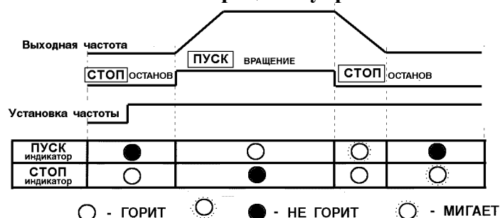
Рис. 11. Пояснения к пульту управления Изменение состояний световых индикаторов "ПУСК" и "СТОП" в процессе управления
